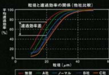
グラフは、スラッジ(異物)の粒径と通過効率の関係を示したもので、 通過効率がノーマル比で最大34%向上していることが認められます。
