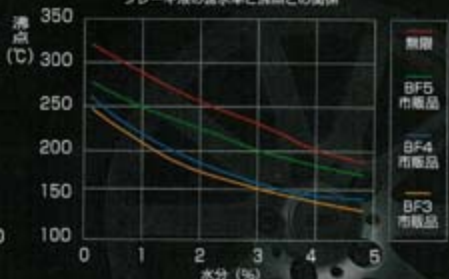
ブレーキ液の含水率と沸点との関係
