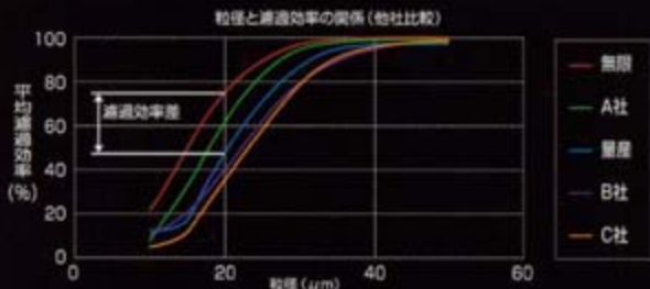
【粒径と通過効率の関係 グラフ】 上のグラフはスラッジ(異物)の粒径と通過効率の関係を示したグラフです。 通過効率が量産比で最大36%向上している事が認められます。
