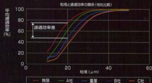
【粒径と通過効率の関係 グラフ】
