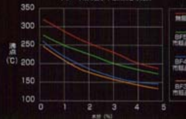
ブレーキ液の含水率と沸点との関係
