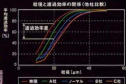
グラフは、スラッジ(異物)の粒種と濾過効率の関係を示したもので、濾過効率がノーマル比で最大36%向上していることが認められます。
