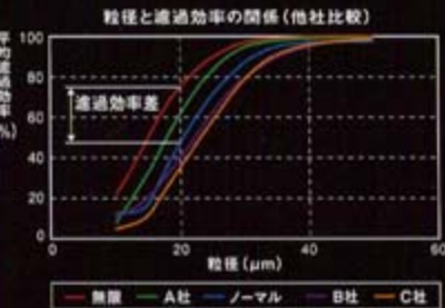
グラフは、スラッジ(異物)の粒径と透過効率の関係を示したもので、透過効率がノーマル比で最大36%向上していることが認められます。
