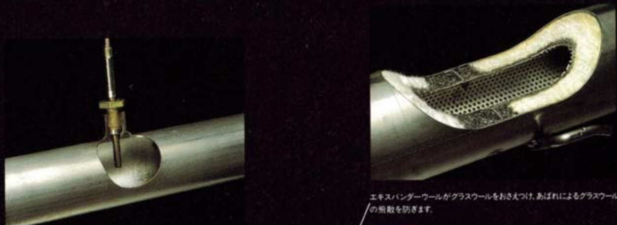
キャクライザー用の温度センサーを装着するためのセンサーホールです。
