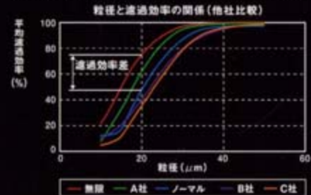
グラフは、スラッジ (異物) の粒径と濾過効率の関係を示したものです。濾過効率がノーマル比で最大36%向上していることが認められます。
