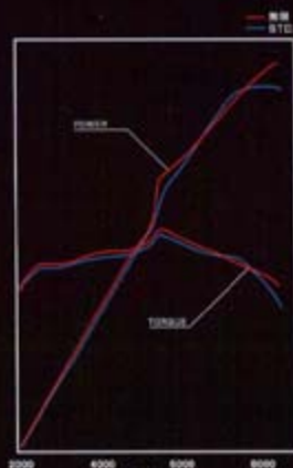
グラフはノーマル状態と無限仕様(ハイパフォーマンスエアクリーナー&ボックス、エキゾーストマニホールド、スポーツエキゾーストシステム装着)を比較したもの。※当社測定値
