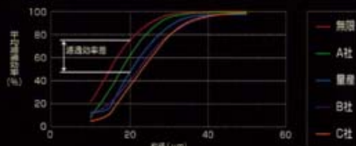
【粘滞と透過効率の関係 グラフ】 上のグラフはスラッジ (異物) の粘滞と透過効率の関係を示したグラフです。透過効率が量産比で最大35%向上している事が認められます。
