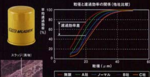
グラフは、スラッジ(異物)の粒径と濾過効率の関係を示したもので、濾過効率でノーマル比で最大36%向上していることが認められる。
